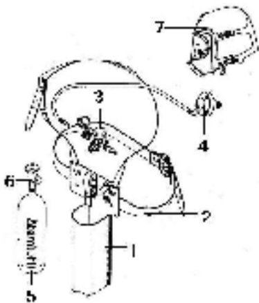
Bild 29: Druckluftselbstretter
