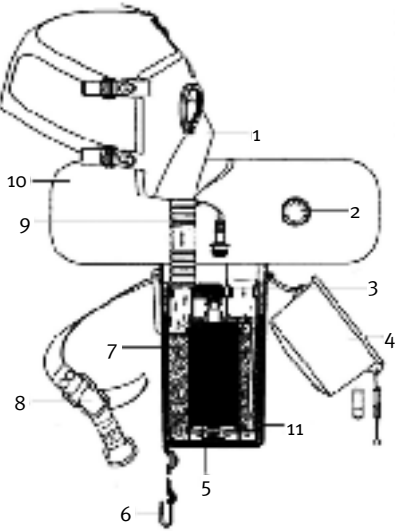
Bild 32: Chemical-Sauerstoff(NaClO 3 )selbstretter
